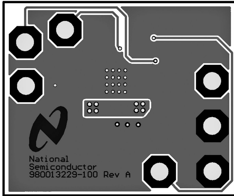
Bottom Layer
